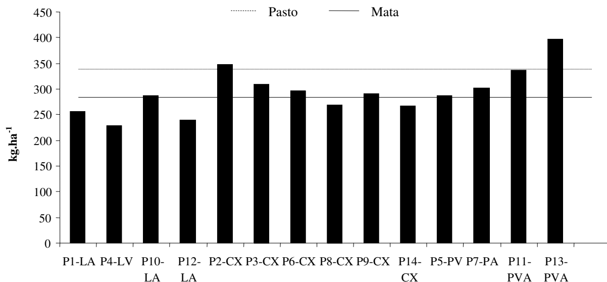
Figura 14: Estoque de K na profundidade de 0,50 m para as áreas estudadas no projeto RECA em Nova Califórnia-RO.
