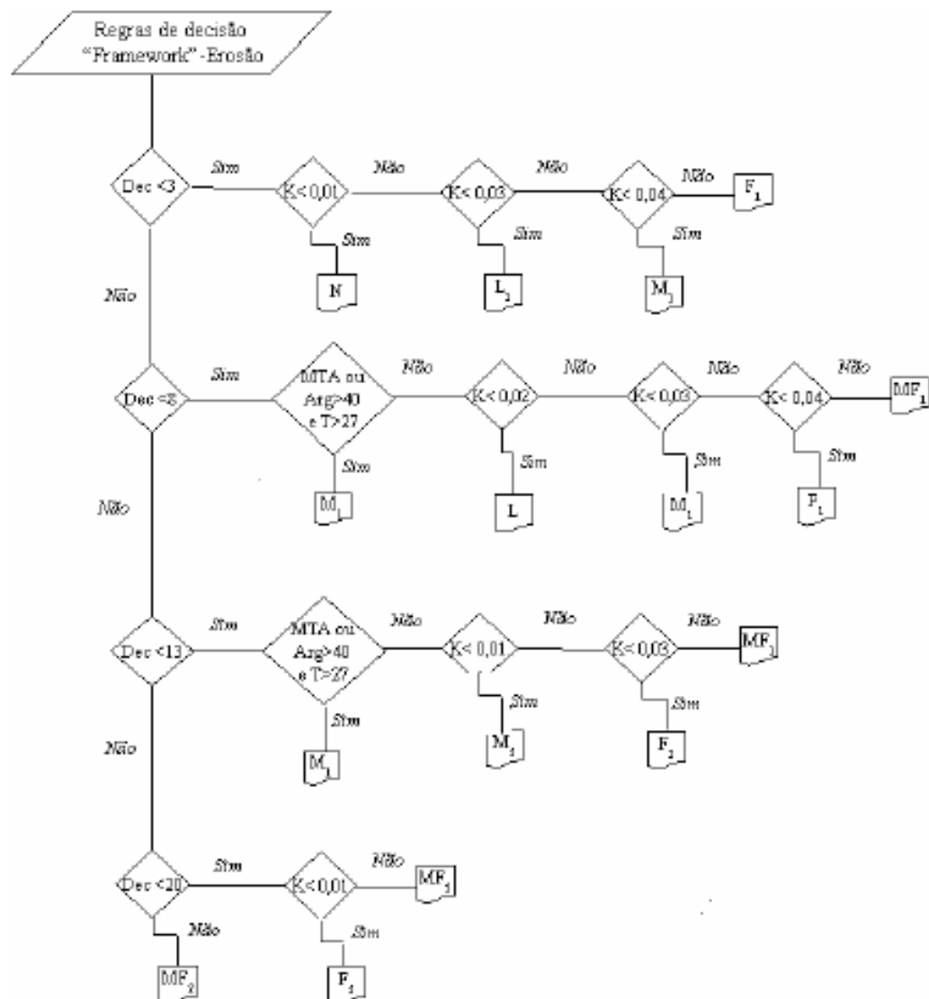
Figura 21: Regras de decisão para determinação do grau de limitação quanto à suscetibilidade à erosão (fonte: Nóbrega et al., 2008b).
