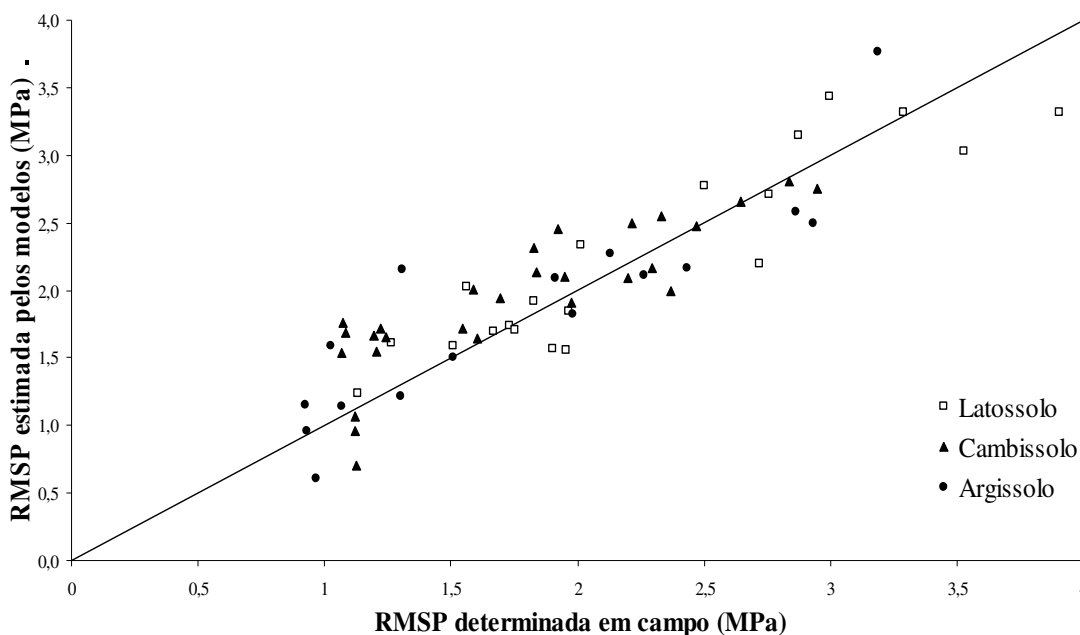
Figura 9: Correlação entre a RMSP determinada e calculada em três ordens de solos sob SAFs do Projeto RECA em Nova Califórnia –RO.
