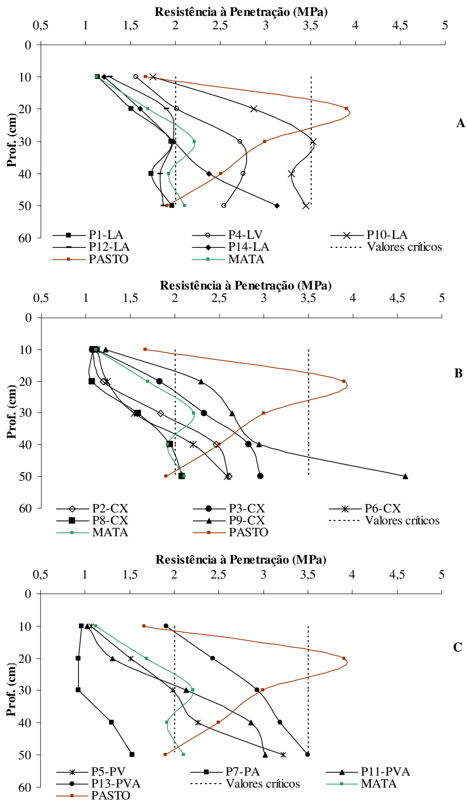
Figura 8: Valores de resistência à penetração em Latossolos (A), Cambissolos (B) e Argissolos (C). Testes realizados em áreas de propriedades do RECA em Nova Califórnia –RO.
