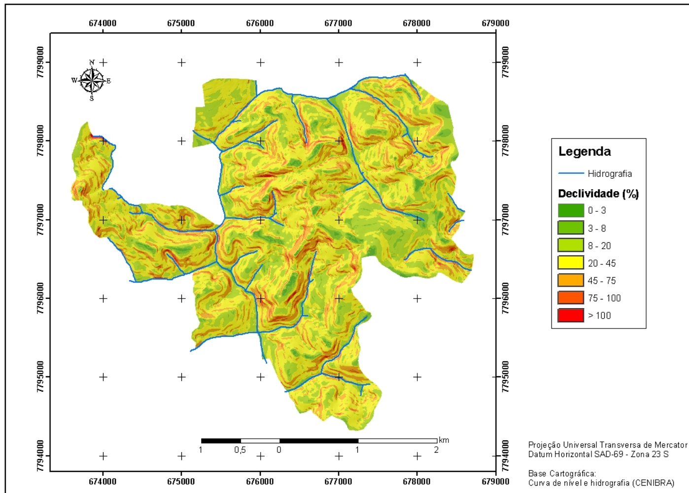
Figura A5. Distribuição das classes de declividade no projeto Florália.
