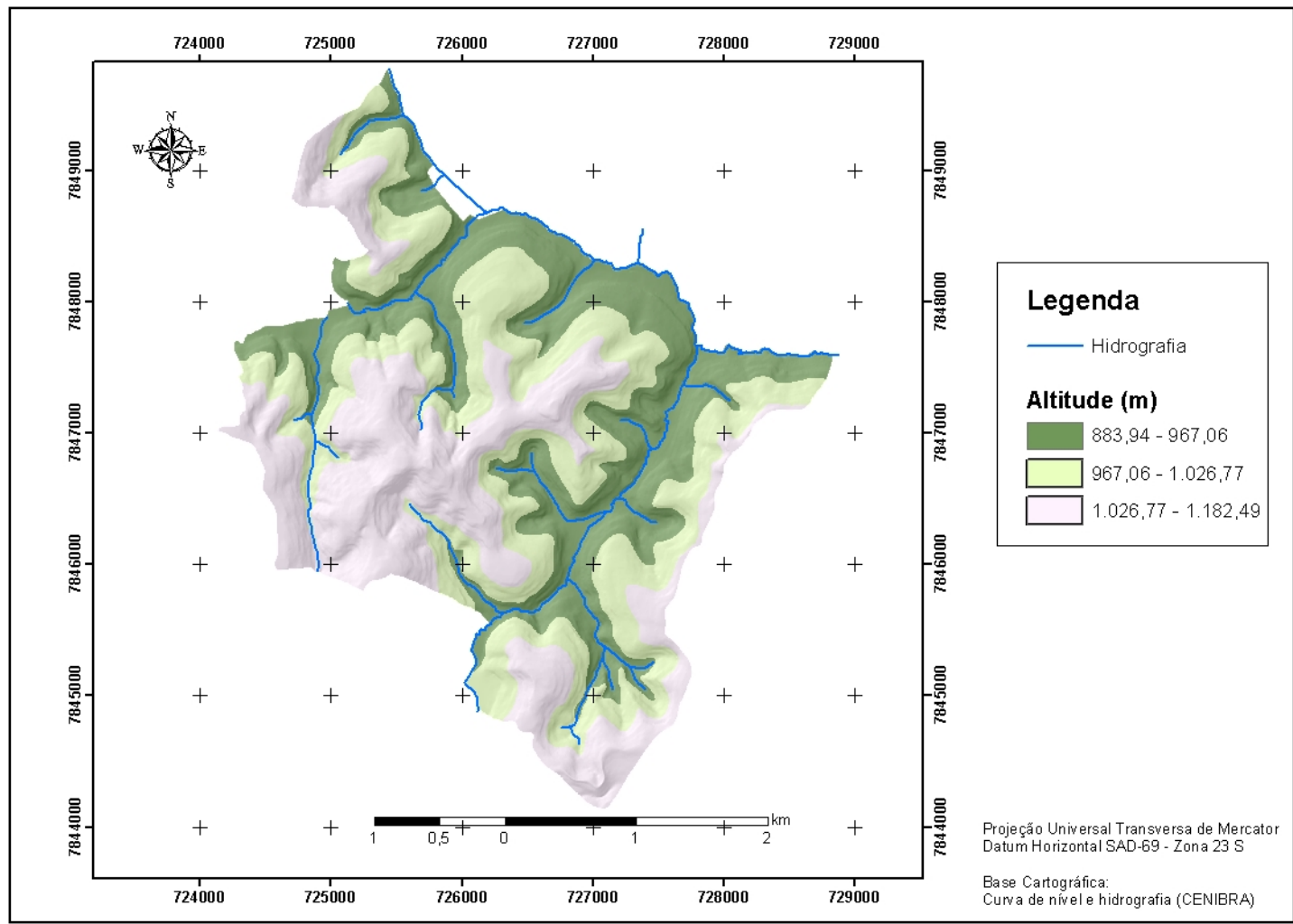
Figura A2. Modelo Digital de Elevação do projeto Jatobá I.
