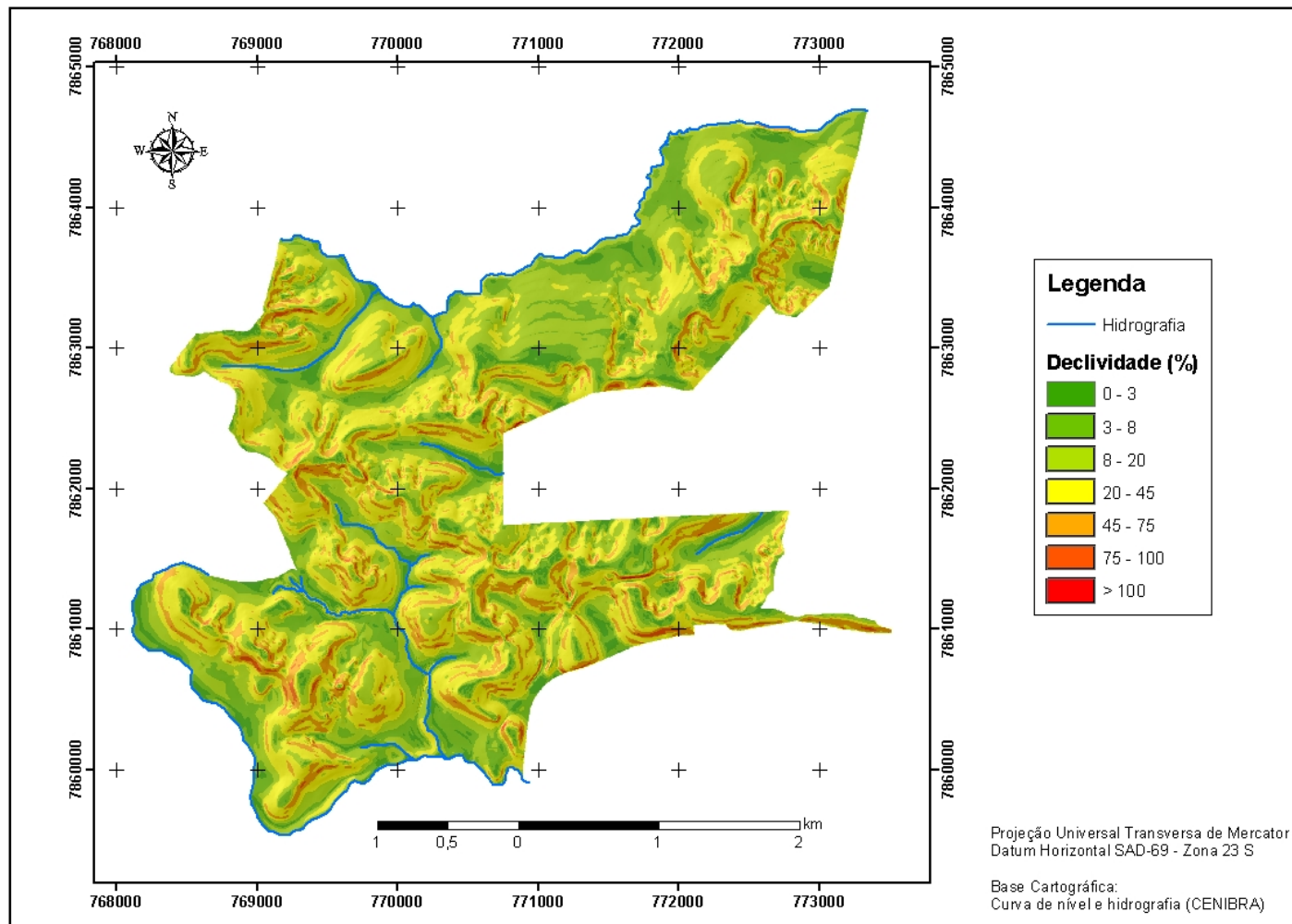
Figura A7. Distribuição das classes de declividade no projeto Marola.
