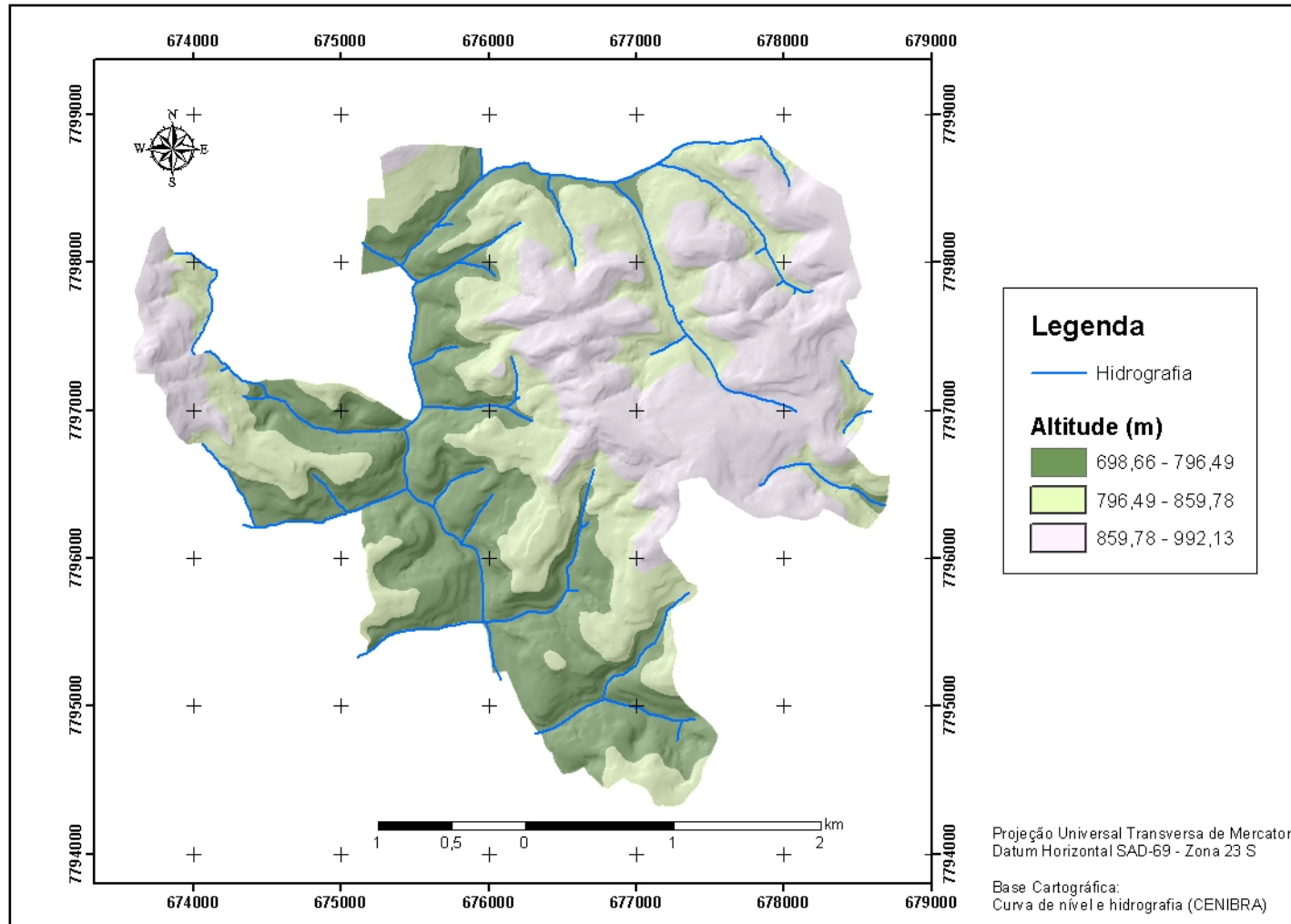
Figura A1. Modelo Digital de Elevação do projeto Florália.
