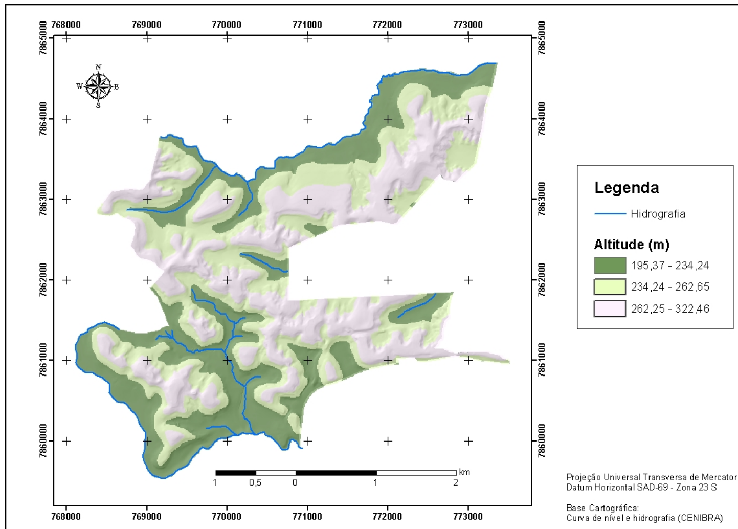
Figura A3. Modelo Digital de Elevação do projeto Marola.
