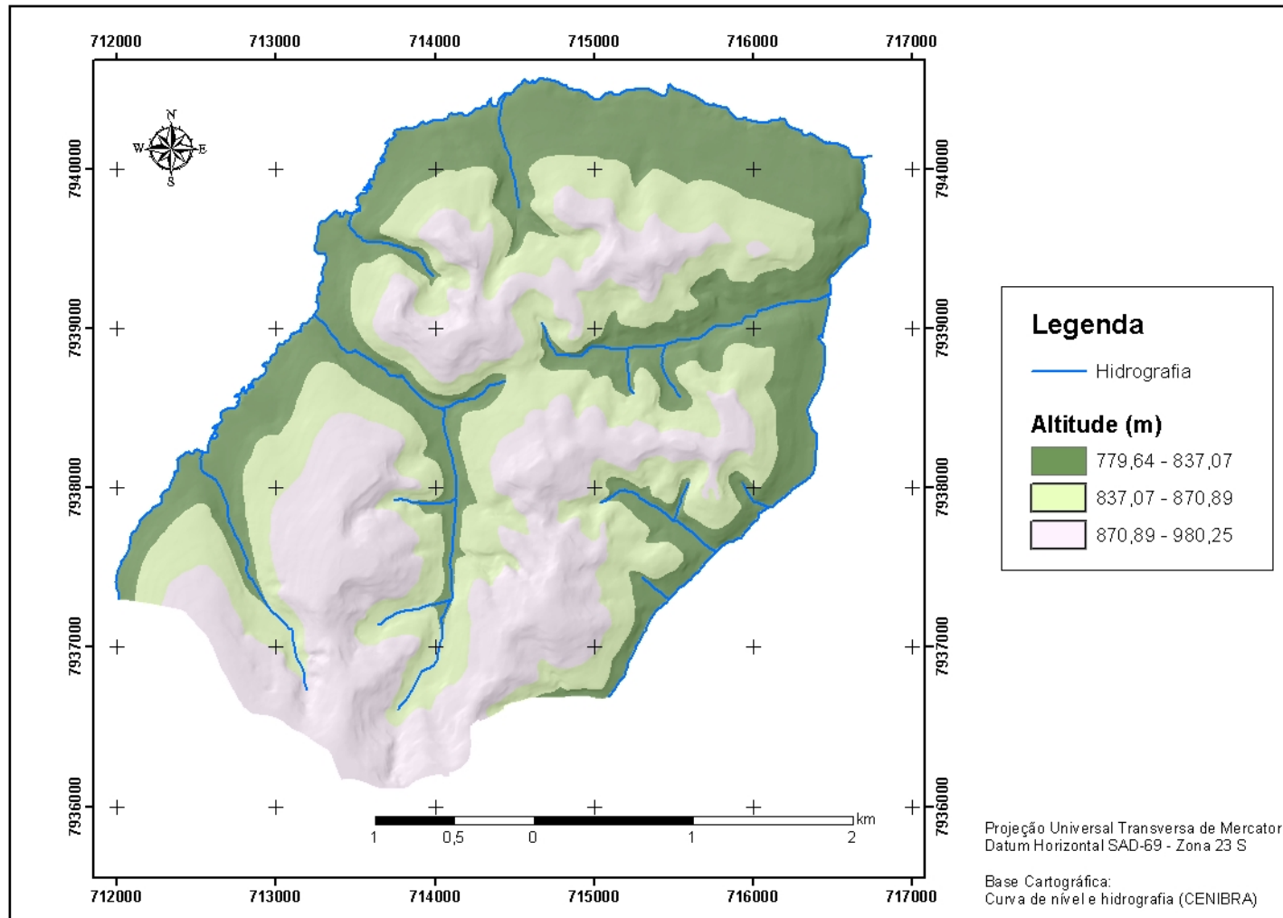
Figura A4. Modelo Digital de Elevação dos projetos Sabinópolis I e III.
