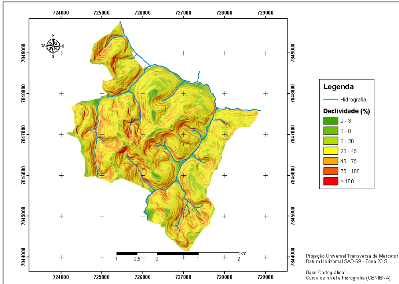
Figura A6. Distribuição das classes de declividade no projeto Jatobá I.
