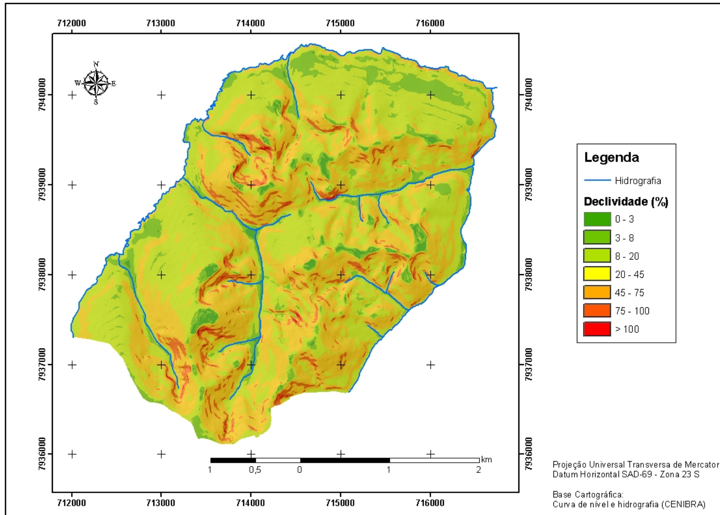
Figura A8. Distribuição das classes de declividade nos projetos Sabinópolis I e III.
