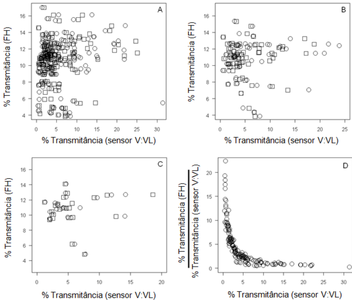
Figura 6. Valores de transmitância com base nas fotografias hemisféricas (FH) e nas medidas do sensor V:VL. Os círculos representam as medidas através do sensor com o baixo esforço amostral e os quadrados as medidas com o alto esforço amostral. (A) Amostras pequenas. (B) Amostras intermediárias. (C) Amostras grandes. (D) Diferença entre as técnicas de estimativas de luz (somente nas amostras pequenas) em função dos valores de transmitância estimados através do sensor com o baixo esforço amostral.
