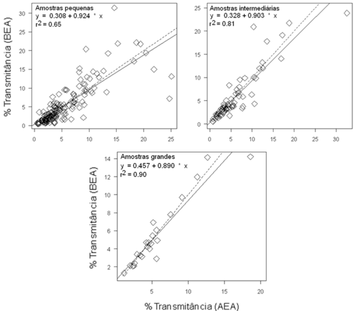
Figura 5. Relação entre a transmitância obtida com o baixo (BEA) e o alto esforço amostral (AEA). A linha tracejada indica aonde os pontos deveriam estar caso não houvesse diferença entre os esforços e a linha contínua representa os valores preditos pelo modelo linear.
