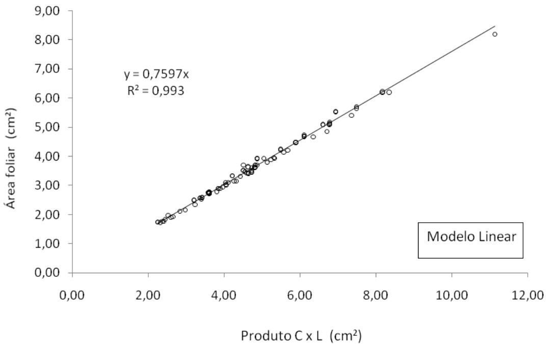
Figura 10 - Correlação entre área foliar ( \text{cm}^2 ) e o produto do comprimento (C) pela largura (L) dos folíolos da Catingueira – modelo linear.
