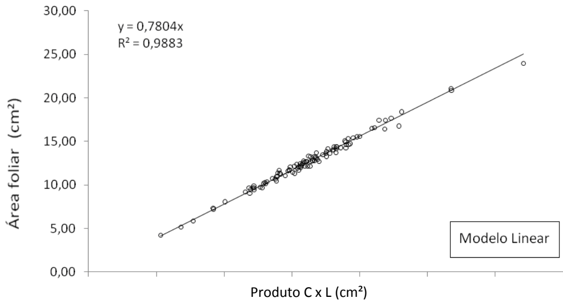
Figura 16 - Correlação entre área foliar ( \text{cm}^2 ) e o produto do comprimento (C) e a largura (L) dos folíolos do Cumaru – modelo linear.
