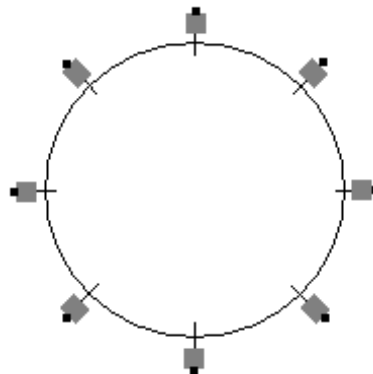
Figura 8. Esquema do posicionamento equidistante e em linha dos sensores na seção transversal do lenho das árvores de teca.
