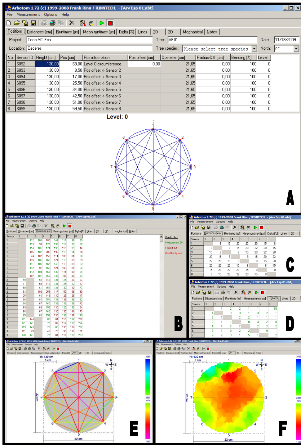
Figura 4. Software ARBOTOM. - (A) Informações fornecidas pelo usuário do Aparelho, como distância entre sensores, medida da circunferência da árvore, informações da espécie, indivíduo e sua localização; (B) Matriz de Runtimes; (C) Distância entre sensores; (D) Matriz de Velocidades; (E) Gráfico de linhas; (F) Gráfico de Superfície.
