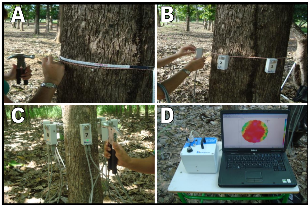
Figura 9. Instalação do tomógrafo de impulso e obtenção das imagens tomográficas. A – Fixação dos condutores metálicos equidistantes; B – Distribuição dos sensores de impulsos; C- Aplicação das pancadas de martelo para produção de ondas mecânicas; D – Imagem tomográfica.
