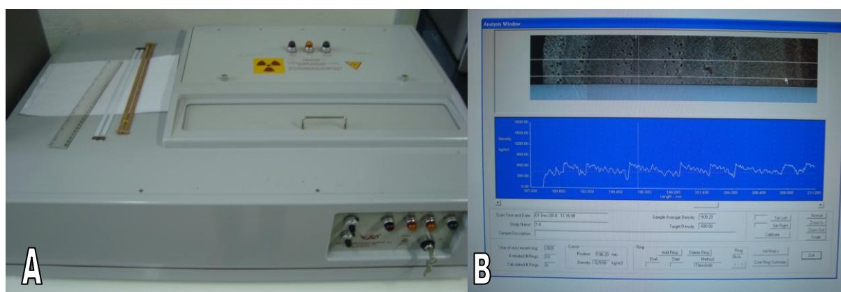
Figura 12. Equipamento utilizado na densitometria de raios X. A - equipamento QTRS-01X Tree-Ring Analyzer; B – Software QMS para obtenção dos perfis radiais de densidade.
