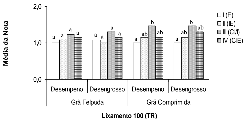
Figura 93. Médias das notas atribuídas aos defeitos obtidos durante o lixamento (100 grana) para a madeira termorretificada em função dos grupos. Médias seguidas de mesma letra não diferem estatisticamente entre si pelo teste de Tukey a 5% de significância.
