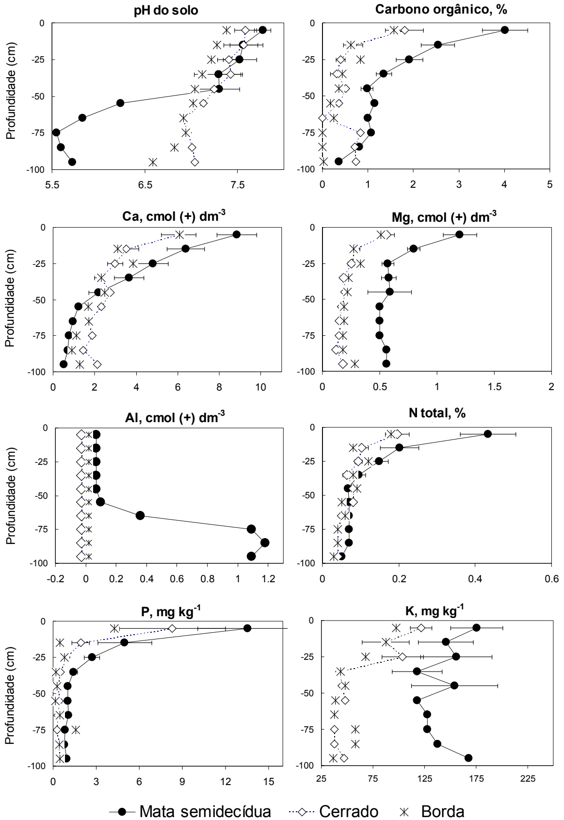
Figura 1.11 – Teor de carbono orgânico, pH do solo, N total, P, K, Ca, Mg e Al disponíveis, em diferentes profundidades do solo, na transição entre mata semidecídua e vegetação aberta de cerrado. Barras de erros representam os desvios-padrão das médias.
