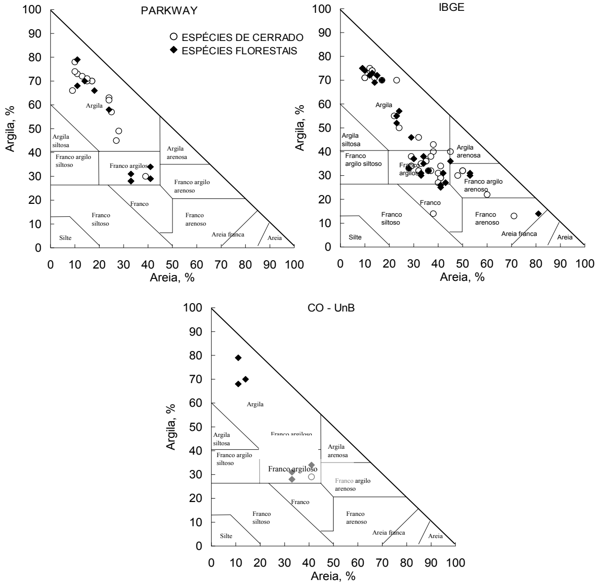
Figura 2.4 – Diagrama de classificação textural dos solos dos três locais de estudo, sob espécies de cerrado e florestais, com base nos percentuais de argila e areia, de acordo com EMBRAPA (1999).
