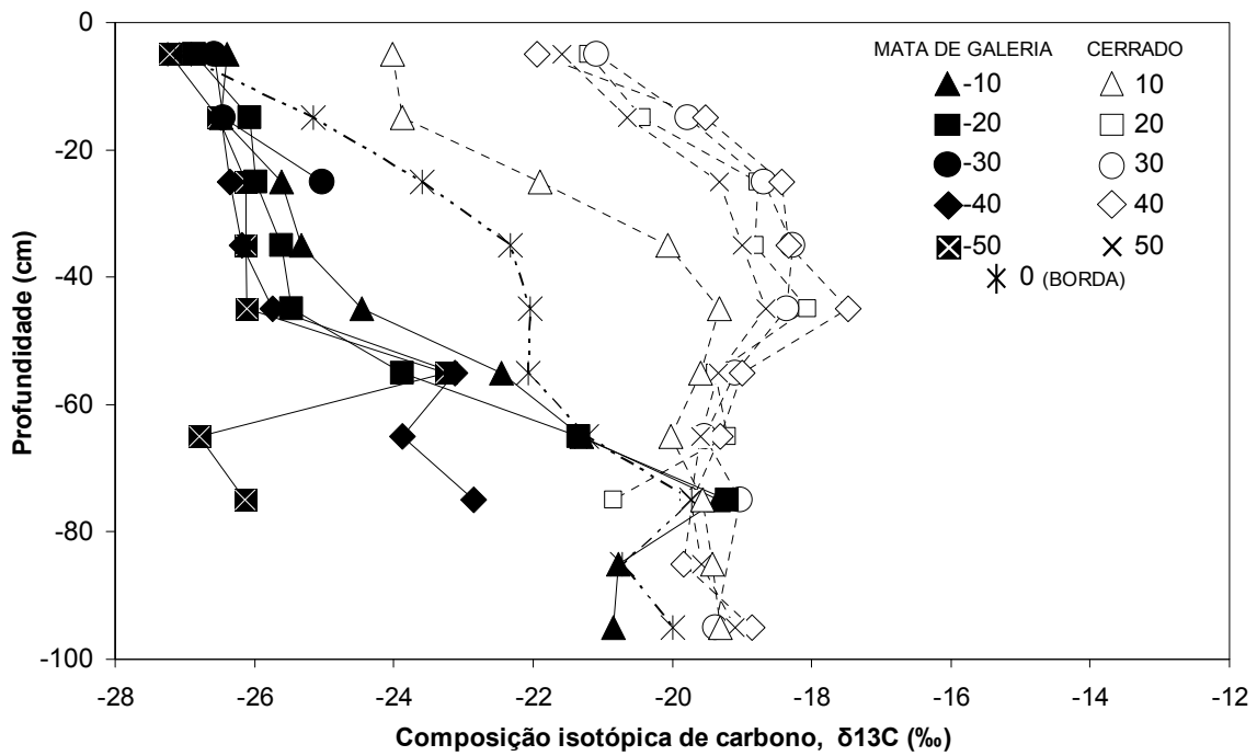
Figura 1.23 - Variação na composição isotópica, \delta^{13}C , em diferentes profundidades do solo, na transição entre cerrado e mata de galeria do Pitoco.
