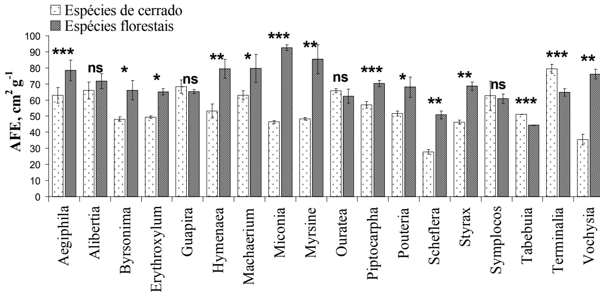
Figura 2.5 – Área foliar específica (AFE) de espécies congêneras características de cerrado e de formações florestais, estabelecidas em áreas de vegetação aberta. Níveis de significância referem-se ao teste t de student, * ( p < 0,05 ), ** ( p < 0,01 ) e ns (diferença não significativa). Barras de erros representam os desvios-padrão das médias.
