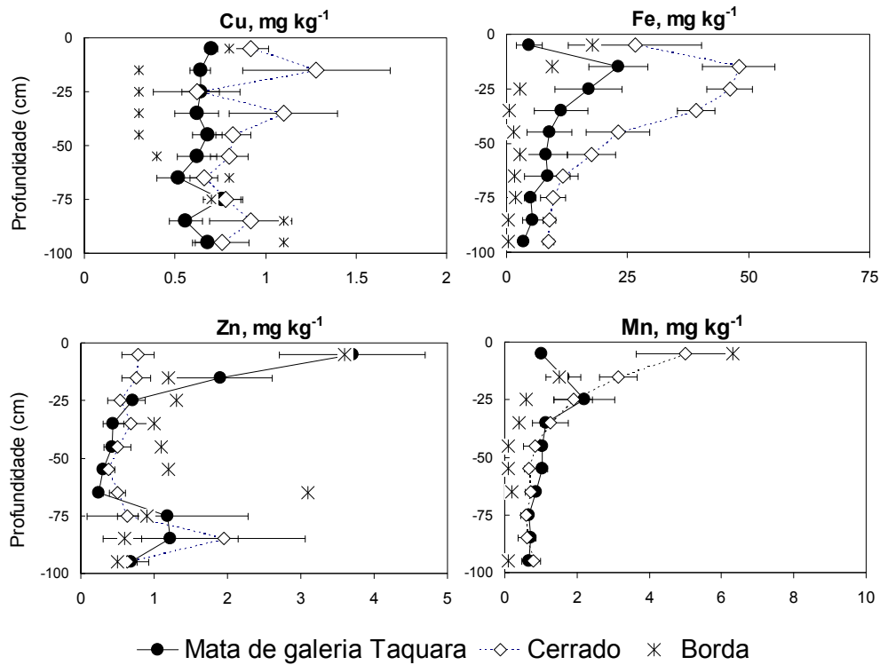
Figura 1.13 - Disponibilidade de Cu, Fe, Zn e Mn em diferentes profundidades do solo, no transecto entre a mata de galeria do Taquara e vegetação aberta de cerrado. Barras de erros representam o desvios-padrão das médias.
