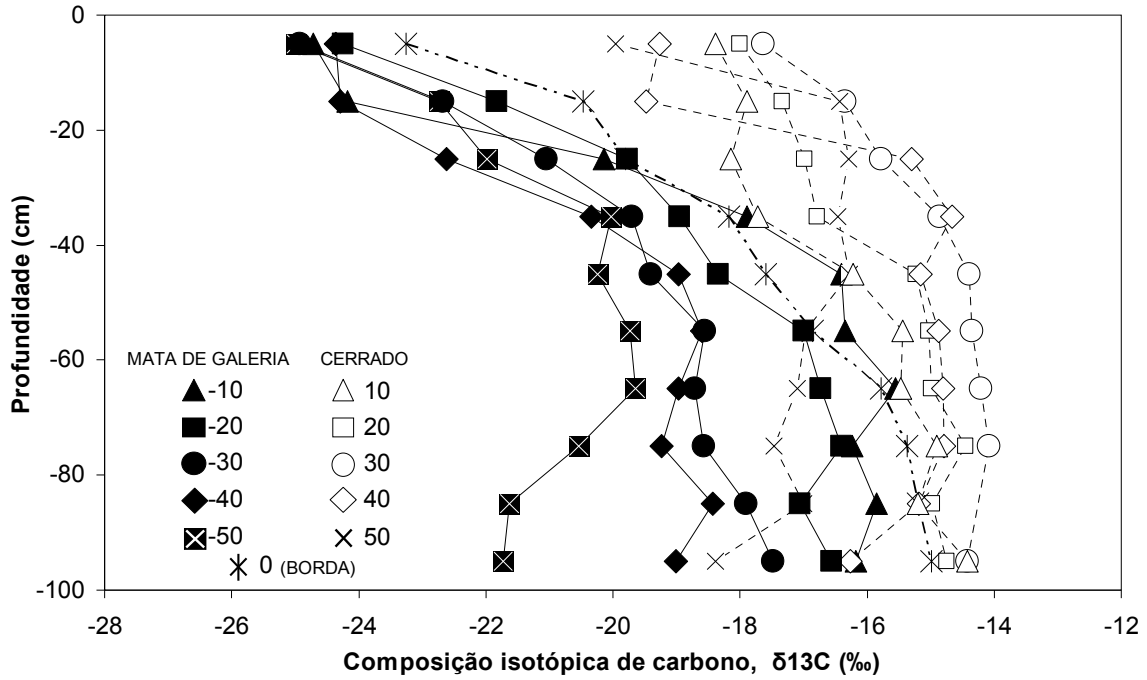
Figura 1.22 – Variação na composição isotópica, \delta^{13}C , em diferentes profundidades do solo, na transição entre cerrado e mata de galeria do Taquara.
