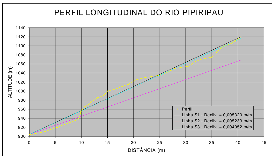
Figura B.1 – Perfil longitudinal do Ribeirão Pipiripau e representação gráfica das linhas S1, S2 e S3 (CAESB, 2001)
