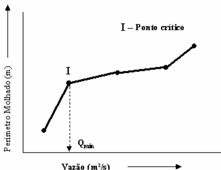
Figura 3.3 – Definição de vazão mínima garantida no método do perímetro molhado a partir do ponto crítico (Loar e Sale, 1981 apud Gonçalves, 2003)
