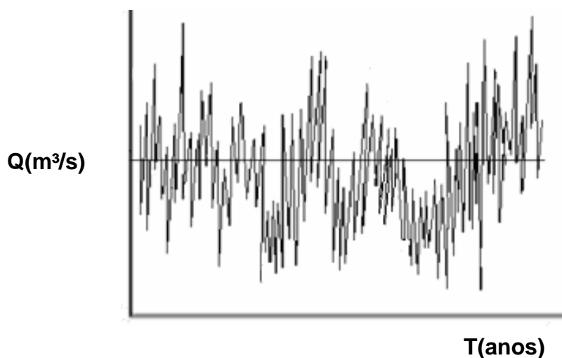
Figura 4.4 – Hidrograma hipotético representando a variabilidade de uma série histórica de vazões.
