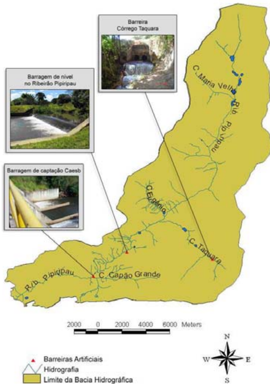
Figura 5.9 – Exemplo de Barreiras Artificiais em trechos da Bacia Hidrográfica do Ribeirão Pipiripau.
