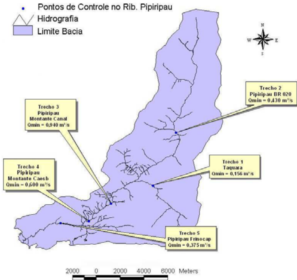
Figura 5.4 – Pontos de controle estabelecidos pela Resolução ADASA nº 293/06 ao longo da Bacia Hidrográfica do Ribeirão Pipiripau e suas respectivas vazões de entrega por trecho
