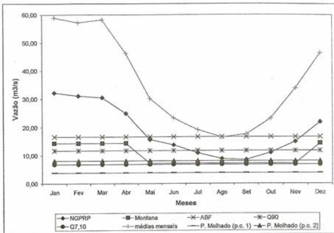
Figura 3.6 Comparação entre os métodos indicados no FTA e vazões médias mensais para o segundo trecho estudado no Rio São Bartolomeu (Gonçalves, 2003)
