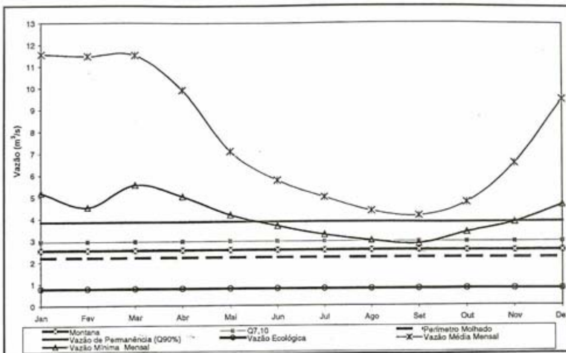
Figura 3.4 Vazões recomendadas para cada mês do ano na aplicação de métodos hidrológicos e hidráulicos recomendados pelo FTA, em trecho à jusante da Barragem do Rio Descoberto (Bezerra, 2001)
