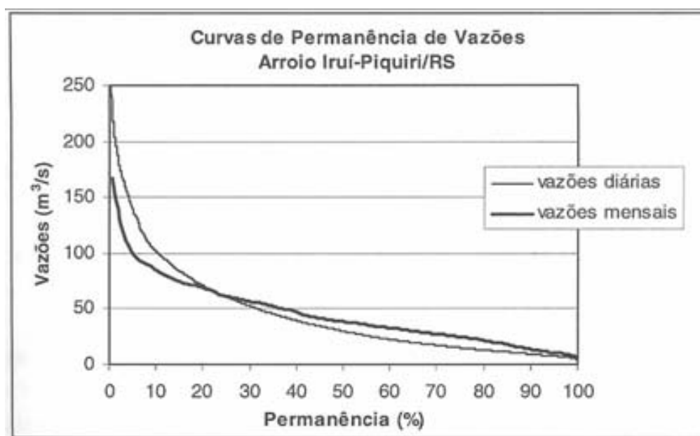
Figura 3.1 – Curvas de permanência de vazões mensal e diária – Arroio Iruí-Piquiri/RS (Silveira e Silveira, 2003).
