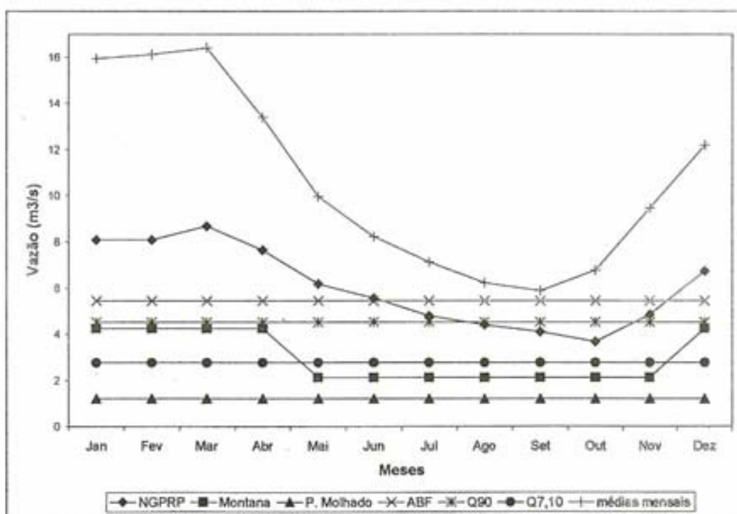
Figura 3.5 Comparação entre os métodos indicados no FTA e vazões médias mensais para o primeiro trecho estudado no Rio São Bartolomeu (Gonçalves, 2003)
