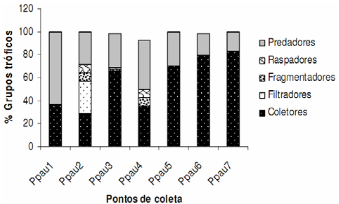
Figura B.3 – Distribuição dos grupos funcionais de alimentação entre os pontos de coleta de macroinvertebrados no Ribeirão Pipiripau (Fernandes, 2007)
