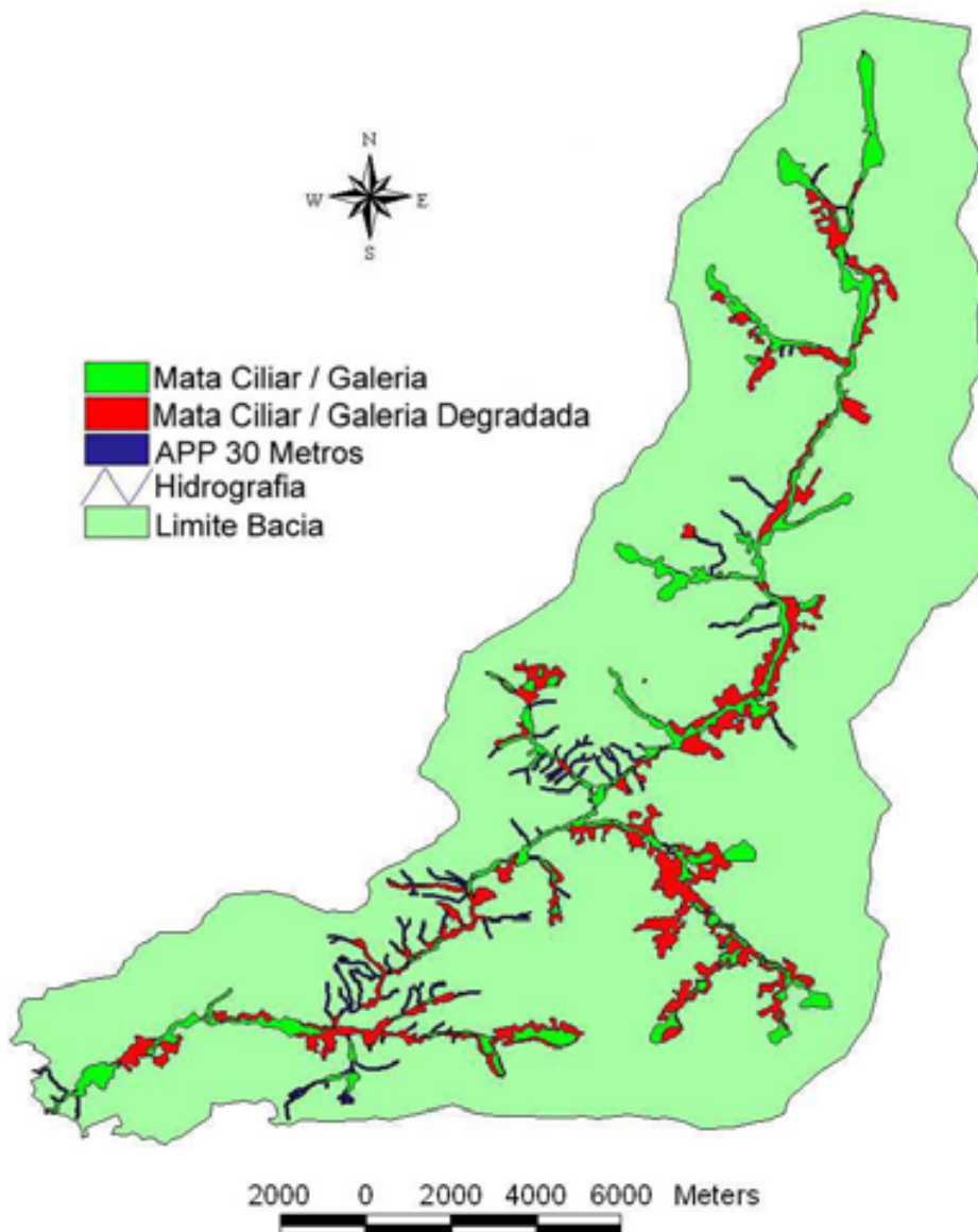
Figura 5.10 – Matas Ciliares e Matas de Galeria ao longo da rede de drenagem da Bacia Hidrográfica do Ribeirão Pipiripau
