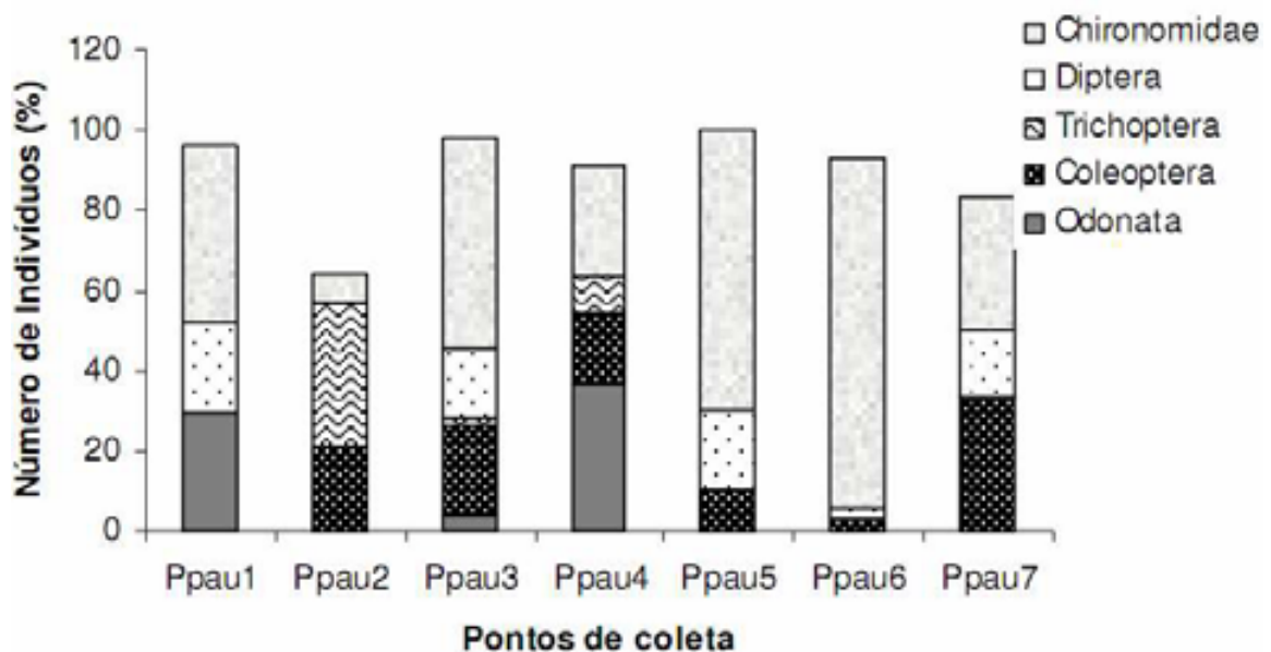
Figura B.2 – Percentagem do somatório do número de indivíduos, no período de seca, nos principais táxons registrados nos diferentes pontos de coleta de macroinvertebrados no Ribeirão Pipiripau (Fernandes, 2007).
