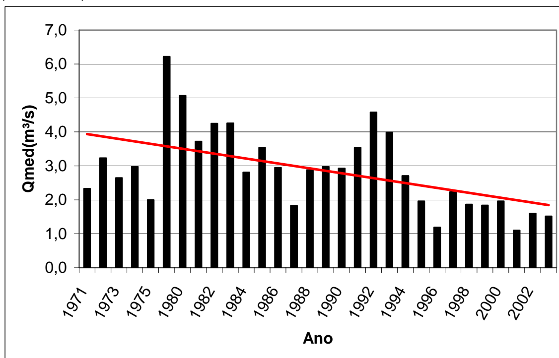
Figura 5.6 – Vazões médias anuais em m³/s no posto FRINOCAP no período (1971-2003)
