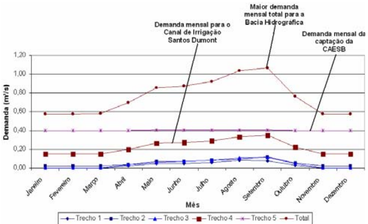
Figura 5.7 – Demandas mensais por trecho na Bacia Hidrográfica do Ribeirão Pipiripau (modificado de ANA, 2004)
