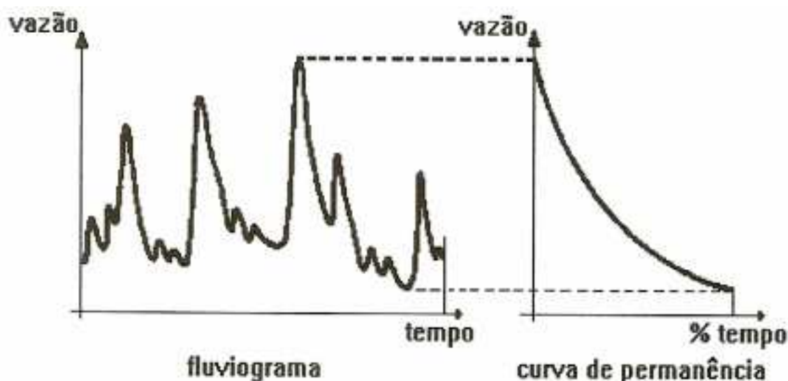
Figura 3.2 – Representação esquemática do fluviograma e respectiva curva de permanência baseada em Quimpo e McNally (1983) apud Cruz (2001).
