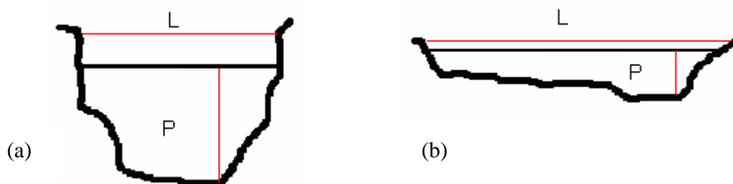
Figura 4.8 – Representação esquemática da razão largura/profundidade em perfil transversal do curso d’água (a) Baixa razão largura/profundidade; (b) Alta razão largura/profundidade.
