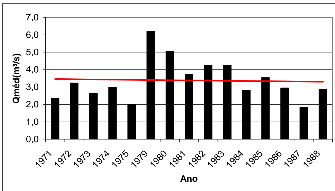
Figura 5.5 – Vazões médias anuais em m³/s no posto FRINOCAP no período (1971-1988)
