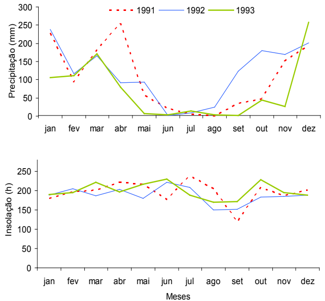
Figura 1. (A) Precipitação (mm) e (B), insolação (horas), ao longo dos anos de acompanhamento fenológico de Protium heptaphyllum . Dados da Estação Agroclimatológica de Nhumirim (SORIANO, 1997).
