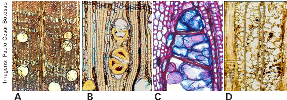
Figura 6. Seção transversal mostrando vasos obstruídos por tilos. A) Cardeiro, ( Scleronema micranthum , Malvaceae); B) ucuúba-punã ( Iryanthera tricornis , Myristicaceae); C) Seringueira ( Hevea brasiliensis , Euphorbiaceae); D) Matamatá, sapucaia cheirosa, tauari ( Eschweilera coriacea , Sin.: E. odora , Lecythidaceae), sendo D em seção longitudinal radial.
