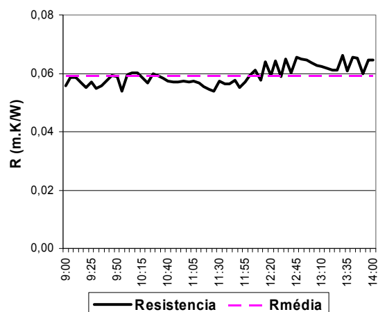
B - CIMENTO-MADEIRA
