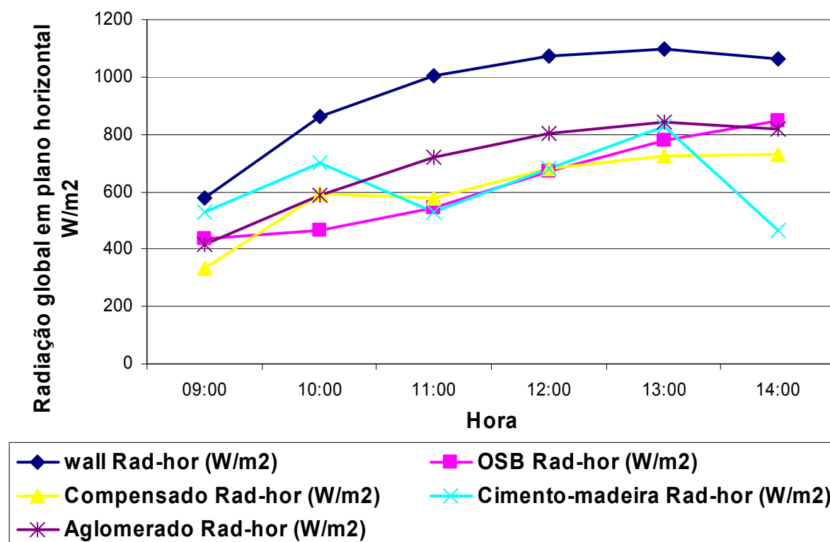
GRÁFICO 16 – COMPARAÇÃO DA RADIAÇÃO GLOBAL EM PLANO HORIZONTAL MEDIDA PRÓXIMA AOS PROTÓTIPOS COM PAINÉIS DE MADEIRA
