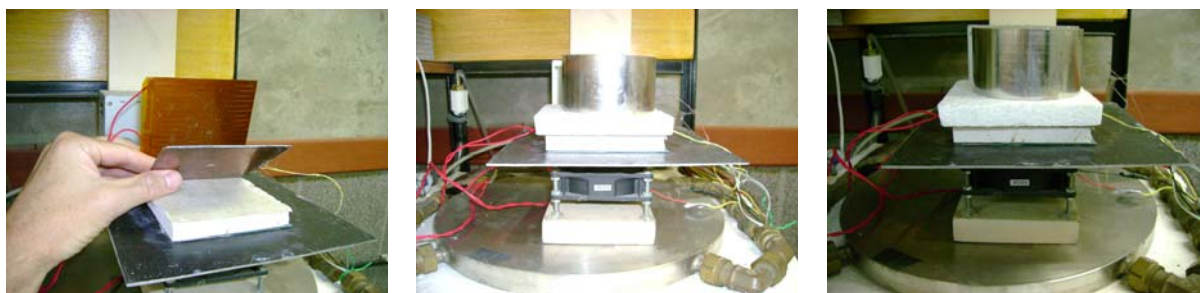
FOTO 45 – FOTOS DO EQUIPAMENTO CONDUTIVÍMETRO FLUXIOMÉTRICO FONTE: LMPT (2008)
