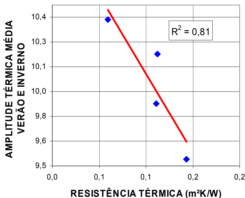
GRÁFICO 25 - RELAÇÃO ENTRE RESISTÊNCIA TÉRMICA E AMPLITUDE TÉRMICA FONTE: KRÜGER ET AL (2008)
