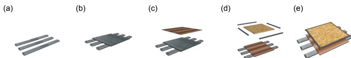
FIGURA 32 – SEQÜÊNCIA DO GRAMPEAMENTO 1 FONTE: O AUTOR (2007)
