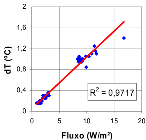
C - COMPENSADO
