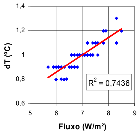
D - OSB
