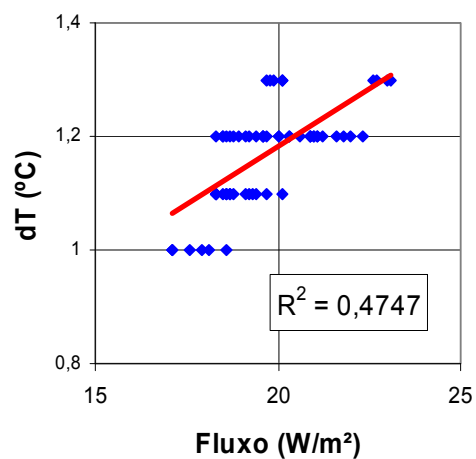
B - CIMENTO-MADEIRA
