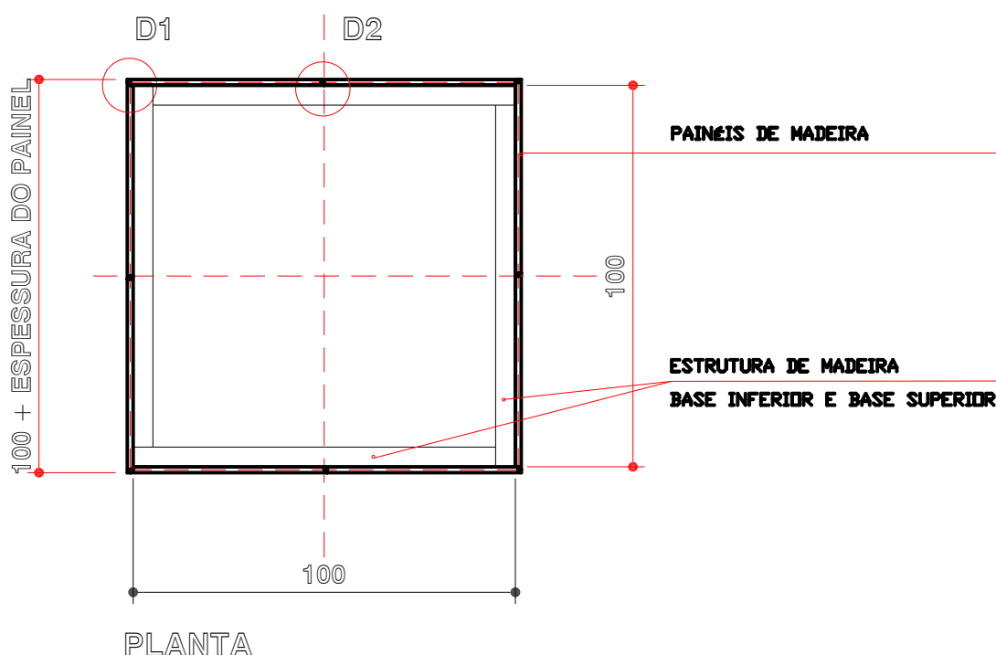
FIGURA 40 – PLANTA DOS PROTÓTIPOS FONTE: O AUTOR (2007)
