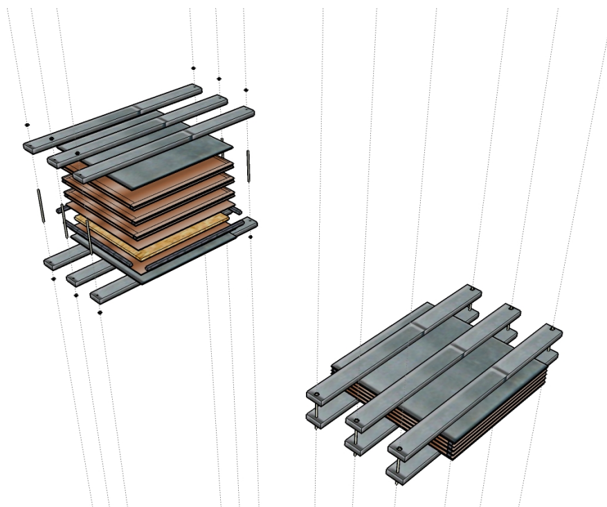
FIGURA 35 - DETALHE DA SEQÜÊNCIA E GRAMPEAMENTO FINAL FONTE: O AUTOR (2007)
