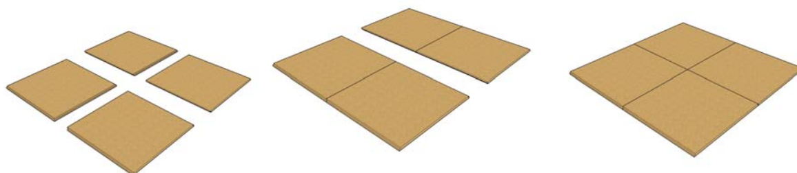
FIGURA 37 POSTERIORMENTE AS DUAS PARTES COLADAS FORMARAM UM DOS PAINÉIS DE VEDAÇÃO LATERAL DO PROTÓTIPO FONTE: O AUTOR (2007)
