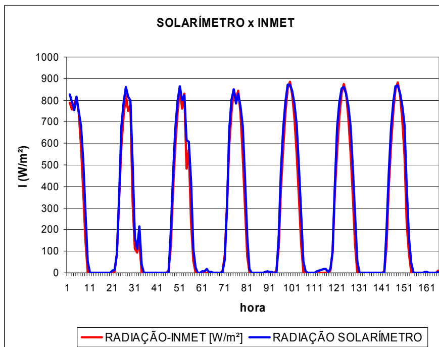
GRÁFICO 6 – COMPARAÇÃO ENTRE DADOS DE RADIAÇÃO MEDIDOS PELO SOLARÍMETRO E DADOS OBTIDOS NO INMET
