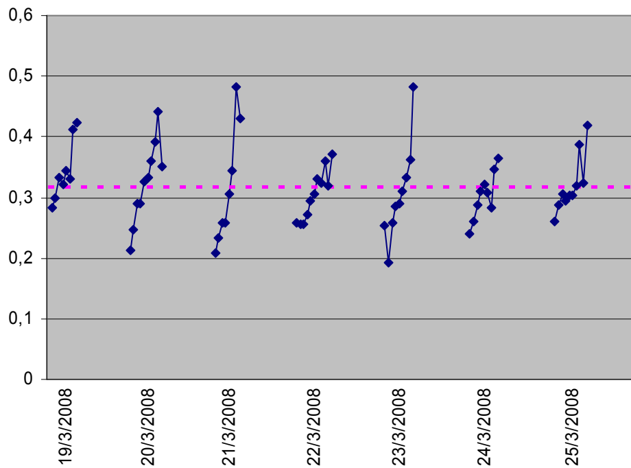
GRÁFICO 9 – VALORES DO ALBEDO PARA OS VÁRIOS DIAS E POSIÇÕES CONSIDERADAS E A TENDÊNCIA DO VALOR MESMO PARA 0,30 FONTE: DO AUTOR (2008)
