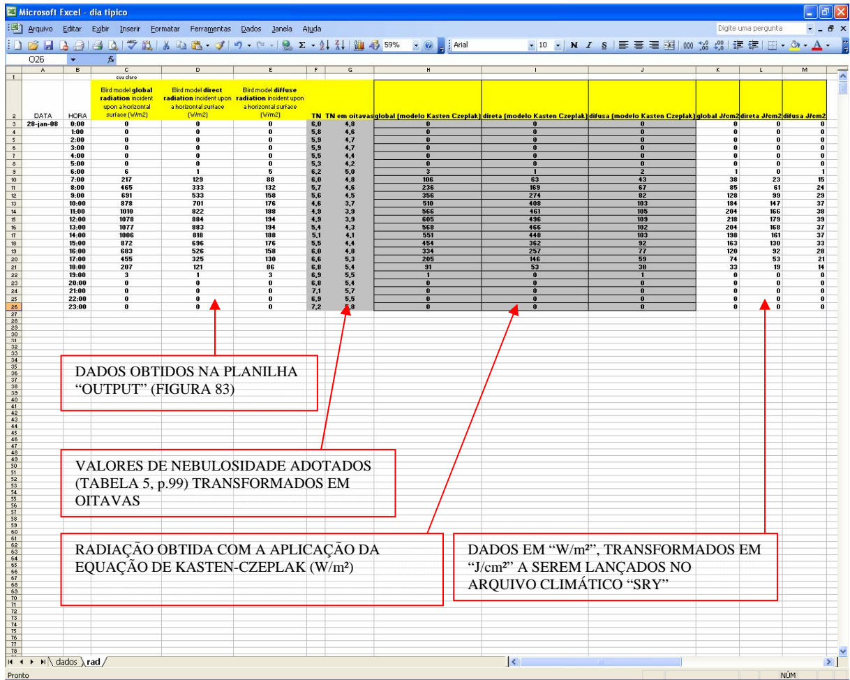
FIGURA 56 – OBTENÇÃO DE RADIAÇÃO GLOBAL EM PLANO HORIZONTAL, RADIAÇÃO DIRETA E RADIAÇÃO DIFUSA FONTE: DO AUTOR (2008)
