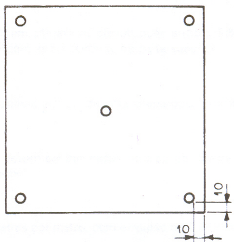
FIGURA 36 - PONTOS DE MEDIÇÃO MARCADAS NOS CORPOS DE PROVA SEGUNDO NORMA ABNT - NBR ABCDE-1 - DIMENSÕES EM MM
