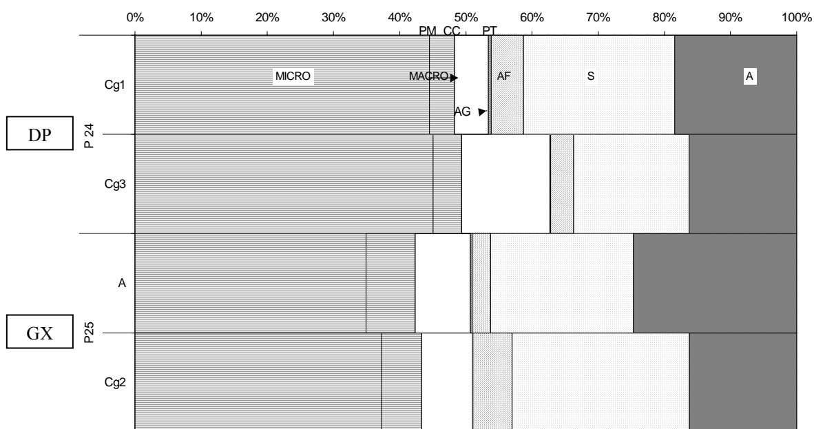
Figura 79 – Distribuição volumétrica das partículas minerais do solo e dos espaços porosos.
