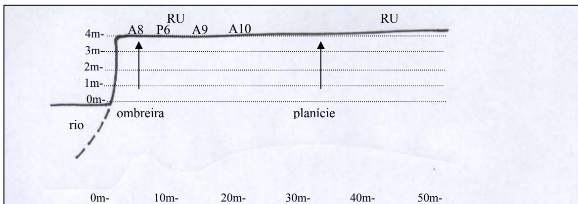
Figura 21 – Corte transversal da superfície de degradação, feições geomórficas, suas dimensões (altura e largura), amostragens e classes de solos.
