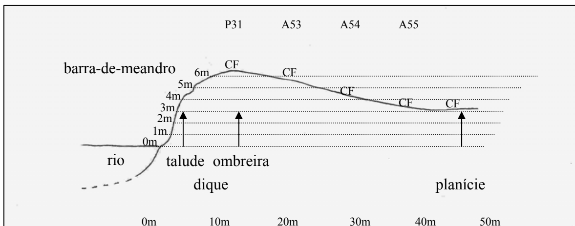
Figura 99 – Corte transversal da superfície de degradação, feições geomórficas, suas dimensões (altura e largura), amostragens e classes de solos.
