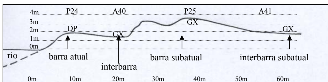
Figura 78 – Corte transversal da superfície de agradação, feições geomórficas, suas dimensões (altura e largura), amostragens e classes de solos.
