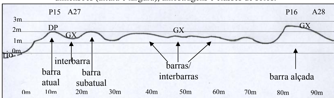
Figura 51 – Corte transversal da superfície de agradação, feições geomórficas, suas dimensões (altura e largura), amostragens e classes de solos.
