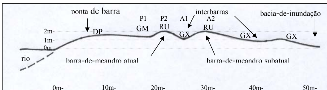
Figura 6 - Corte transversal da superfície de agradação, feições geomórficas, suas dimensões (altura e largura), amostragens e classes de solos.
