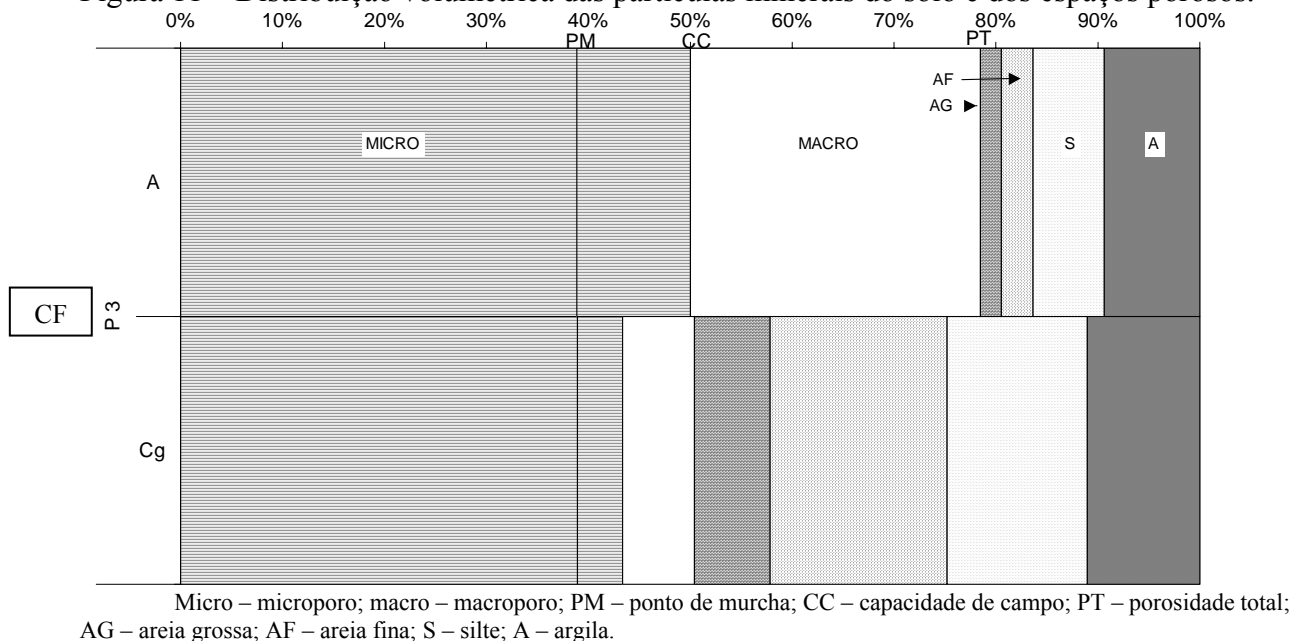
Figura 11 – Distribuição volumétrica das partículas minerais do solo e dos espaços porosos.
