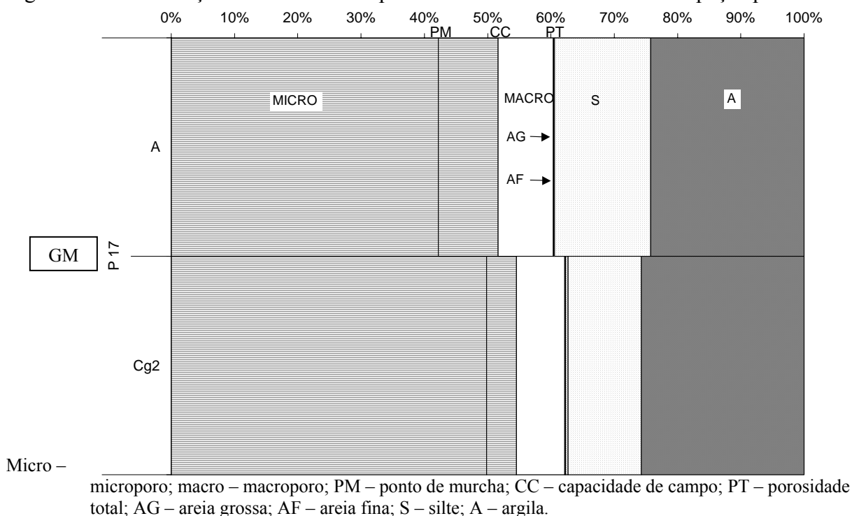
Figura 56 – Distribuição volumétrica das partículas minerais do solo e dos espaços porosos.
