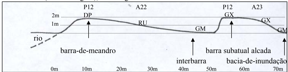
Figura 42 – Corte transversal da superfície de agradação, feições geomórficas, suas dimensões (altura e largura), amostragens e classes de solos.
