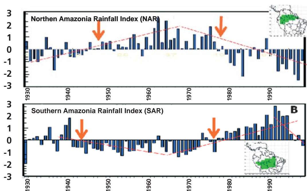
Figura 11. Anomalias normalizadas de chuva para o Norte (a) e para o Sul (b) da Amazônia, desde 1929 a 1997. (Fonte: Marengo, 2004).
