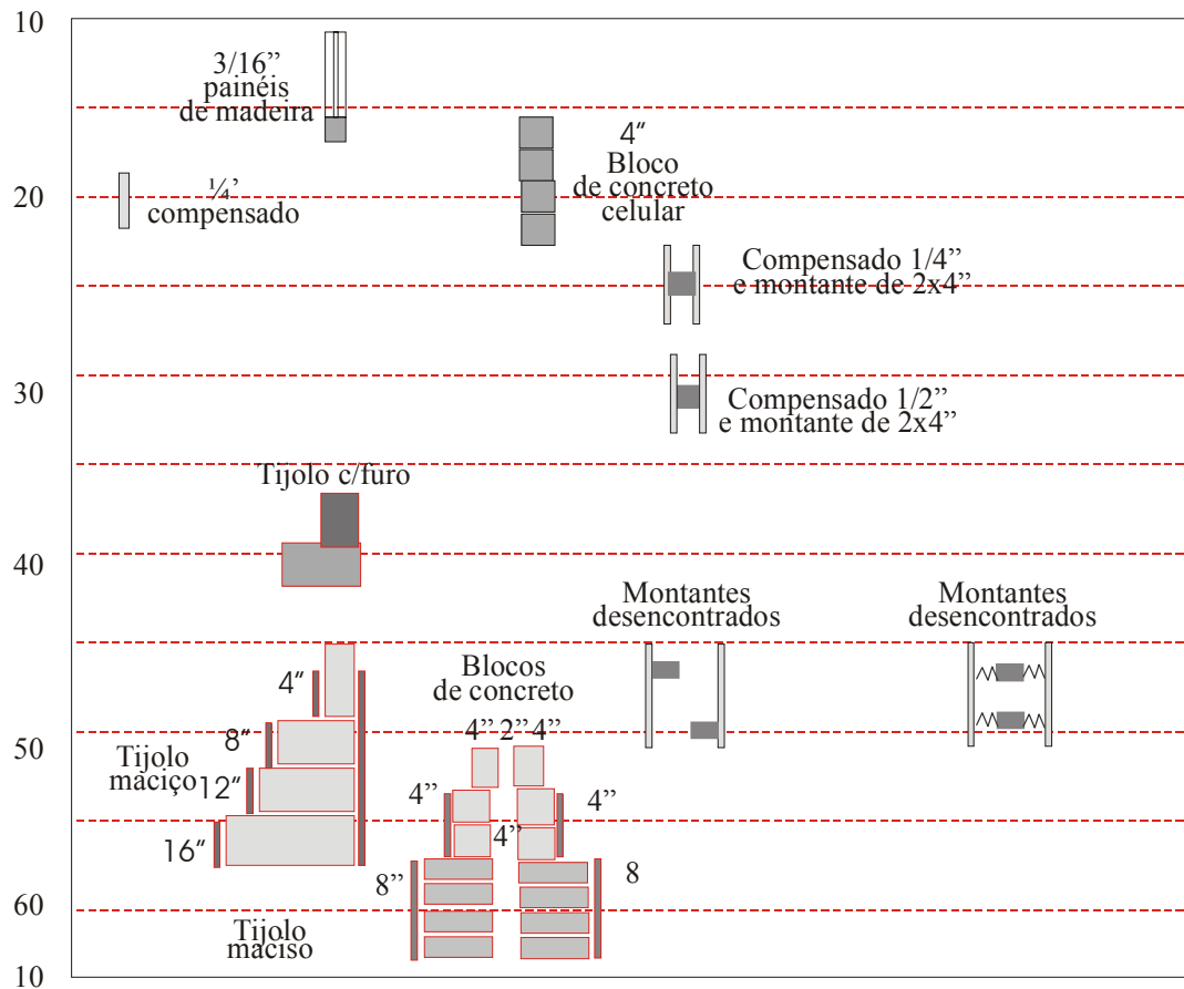
A FIGURA 14- ISOLAMENTO ACÚSTICO DE DIVERSOS MATERIAIS
