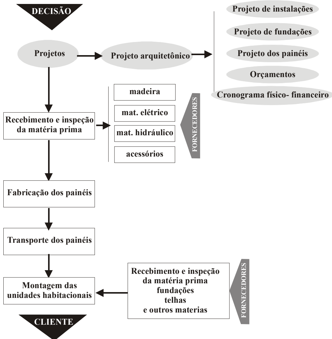
FUGURA28 – FLUXOGRAMA PROCESSO CONSTRUTIVO DO PROTÓIPO
