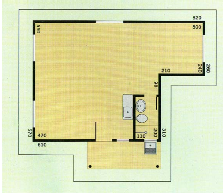
FIGURA 22 -PLANTA BÁSICA – MODELO COHAPAR
