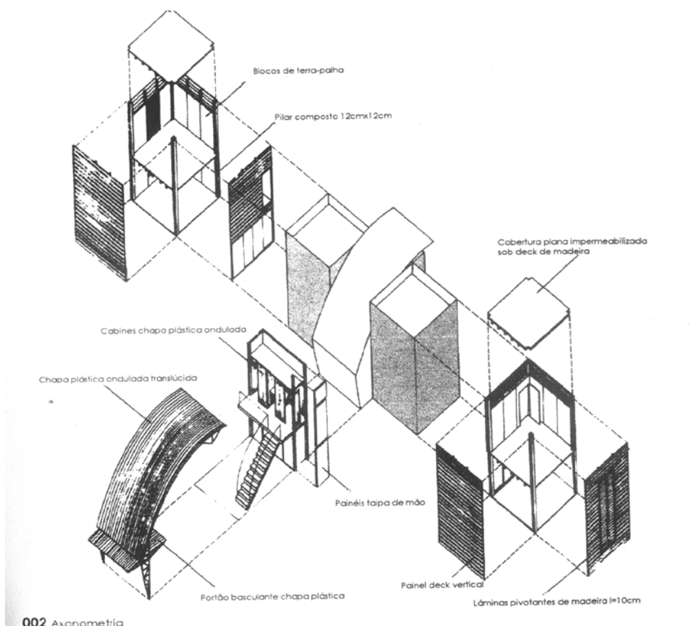
FIGURA 8- HABITAÇÃO SOCIAL EM MADEIRA -UNIDADE 002
