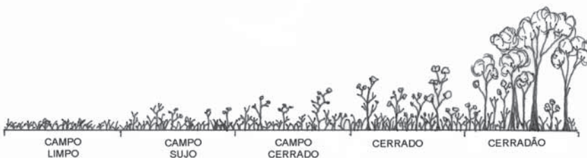
Fig. 2.9 Fisionomias do Cerrado
