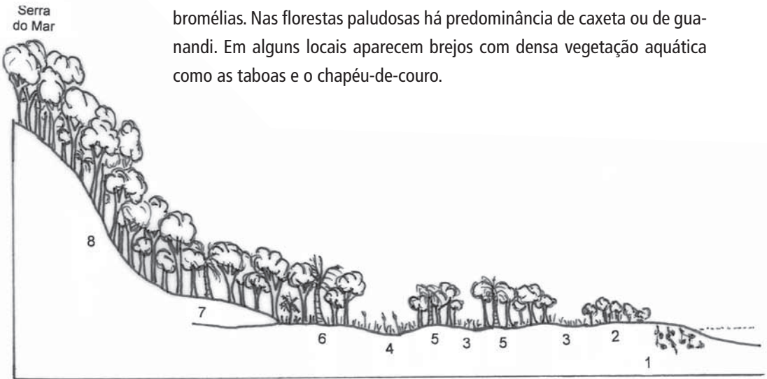
Fig 2.3 Perfil esquemático da Restinga: 1. Vegetação de praia e dunas; 2. Vegetação herbácea, arbustiva/subarbustiva; 3. Vegetação herbáceo-arbustiva em solo encharcado; 4. Brejo; 5. Floresta baixa; 6. Floresta alta; 7. Transição entre restinga e encosta; 8. Mata de encosta
