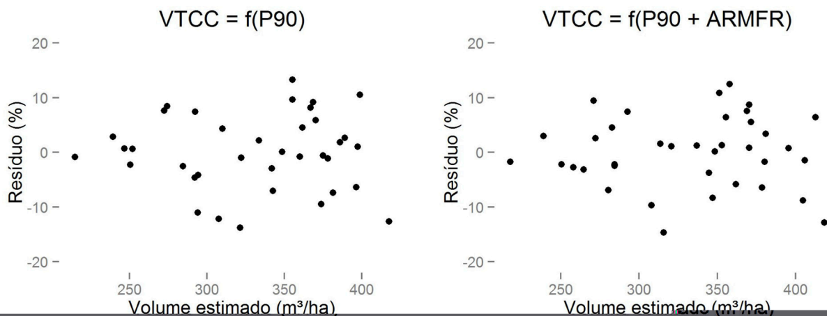
Figura 2. Gráfico percentual dos resíduos em função do volume estimado. Figure 2. Percentage of the residuals related to the estimated volume.
