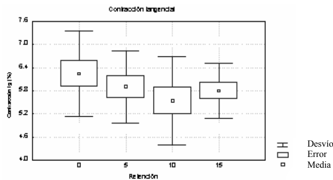
Figura 2. Comparación de medias de contracción tangencial de la madera de Pinus taeda L. sin tratar y tratado con 5, 10 y 15 kg/m 3 .
