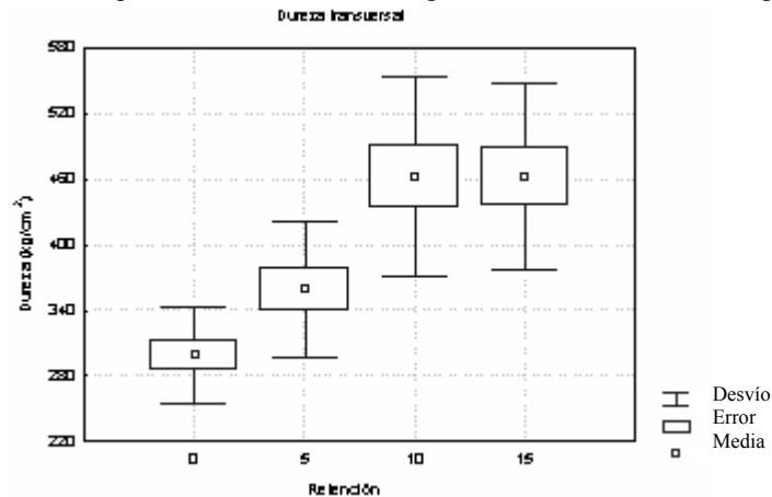
Figura 4. Comparación de medias de dureza Janka transversal de la madera de Pinus taeda L. sin tratar y tratada con 5, 10 y 15 kg/m 3 .
