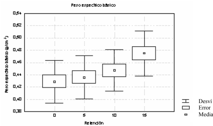
Figura 1. Comparación de medias del peso específico básico de la madera de Pinus taeda L. sin tratar y tratado con 5, 10 y 15 kg/m 3 .
