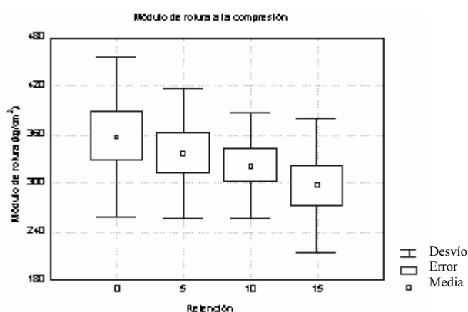
Figura 3. Comparación de medias del módulo de rotura para la compresión paralela a las fibras de la madera de Pinus taeda L. sin tratar y tratada con 5, 10 y 15 kg/m 3 .
