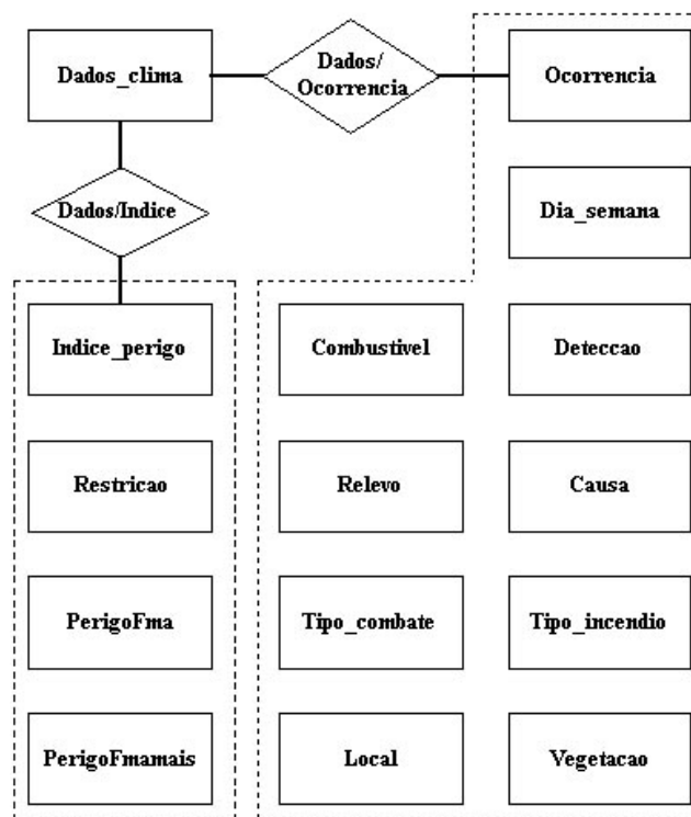
Figura 5. Diagrama de Entidade-Relacionamento.
