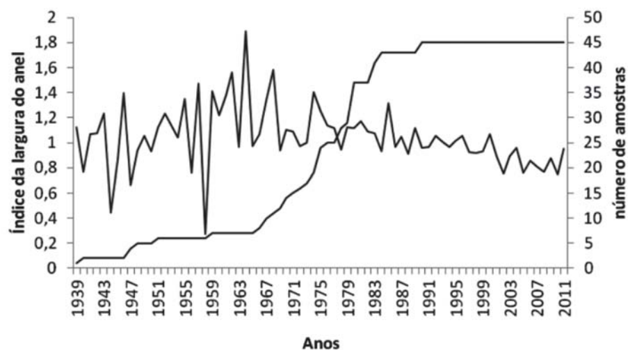
Figura 3 – Série cronológica do índice de largura dos anéis de crescimento do lenho de Schizolobium parahyba e profundidade de série para o conjunto de árvores.
