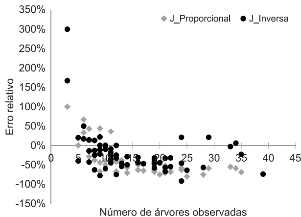
FIGURA 4 Desvio percentual na estimativa do número de árvores pelos métodos da janela proporcional (J_Proportional) e da janela inversa (J_Inversa) em função do número observado de árvores.
