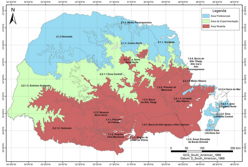
Figura 1. Zoneamento climático para P. caribaea var. hondurensis .
