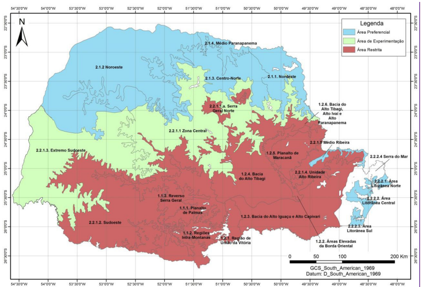
Figura 2. Zoneamento climático para P. caribaea var. caribaea e P. caribaea var. hondurensis .
