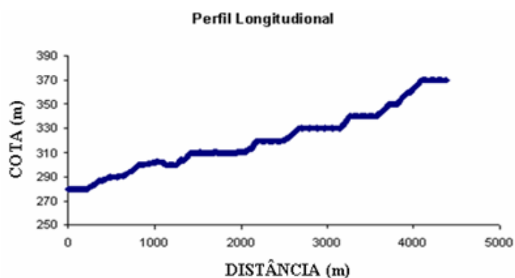
Figura 4. Gráfico do perfil longitudinal da Sub-Bacia Jardim Novo Horizonte, Ilha Solteira, SP (QUEIROZ, 2008).
