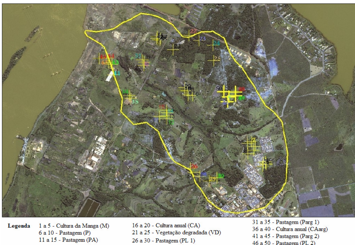
Figura 6. Localização dos pontos de coletas de solo e de avaliações de infiltração e de condutividade hidráulica dos solos.
