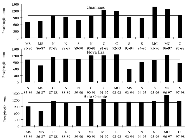
Figura 4 – Precipitação total em cada estação chuvosa, outubro a março, no período de 1985 a 1998, e sua classificação, segundo a técnica dos quantis, para Guanhães, Nova Era e Belo Oriente. A linha cheia representa a média e os símbolos MS, S, N, C e MC, muito seco, seco, normal, chuvoso e muito chuvoso, respectivamente.
