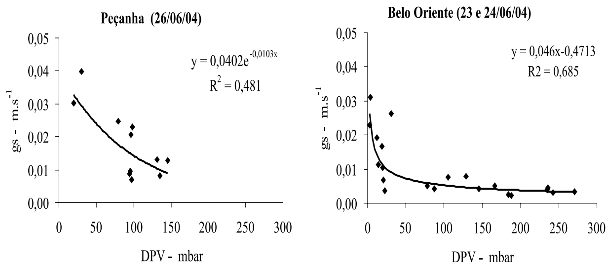
Figura 7 – Condutância estomática ( gs ), m.s^{-1} , e déficit de pressão de vapor (DPV), mbar, em duas regiões da CENIBRA. Figure 7 – Stomatic conductance ( gs ), m.s^{-1} , vapor pressure deficit (VPD), mbar, in two CENIBRA regions.
