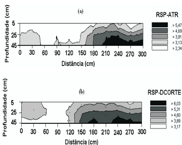
Figura 4 – Mapa de isolinhas da RSP na seção transversal da trilha: antes do tráfego (ATR) (a) e depois do corte (DCORTE) (b).
