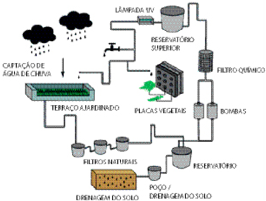
FIGURA 36 – SISTEMA DE REUTILIZAÇÃO DE ÁGUA DE CHUVA. FONTE: TRIPTYQUE ARQUITETURA. (ILUSTRAÇÃO: DIEGO VERNILLE DA SILVA)
