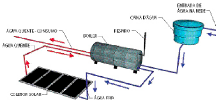
FIGURA 6 – SISTEMA DE AQUECIMENTO DE ÁGUA POR MEIO DE COLETORES SOLARES. UM BOM MAPA-RELHO DE VETERINA ÚTIL DE, NO MÍNIMO, 20 A 30 ANOS. (ILUSTRAÇÃO: NATÁLIA MAYUMI UZUMI)
