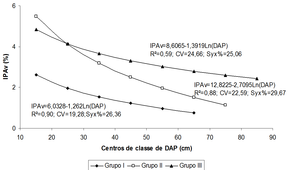
FIGURA 1: Ajuste da curva do incremento periódico anual percentual em volume relacionado ao DAP, para os grupos I, II e III.
