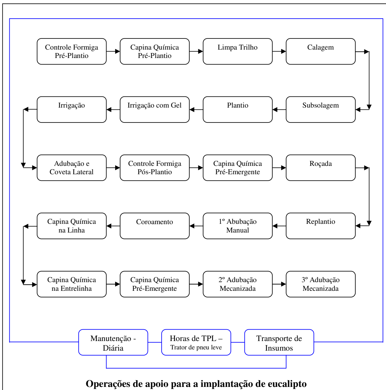
Figura 3. Operações realizadas na implantação de eucalipto.
