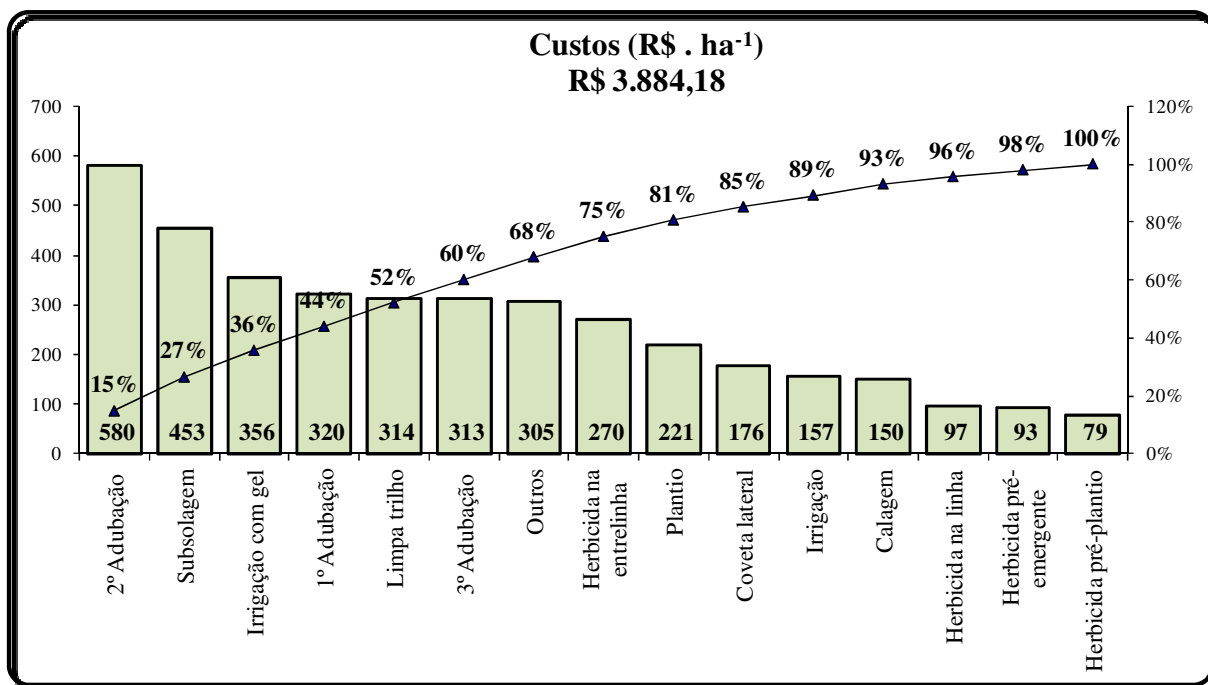
Figura 7. Dispêndios econômicos por operação da implantação de eucalipto. Fonte: Dados da pesquisa de campo (2008/ 2009).
