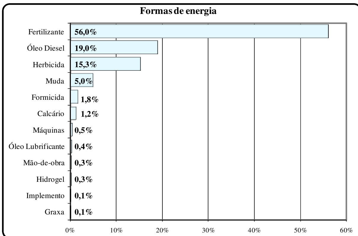
Figura 6. Participação, por ha, das diversas formas de energia na implantação de eucalipto. Fonte: Dados da pesquisa de campo (2008/ 2009).
