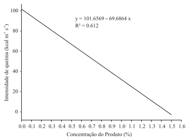
Figura 2 – Intensidade de queima (kcal.m -1 .s -1 ) em diferentes concentrações do produto.
