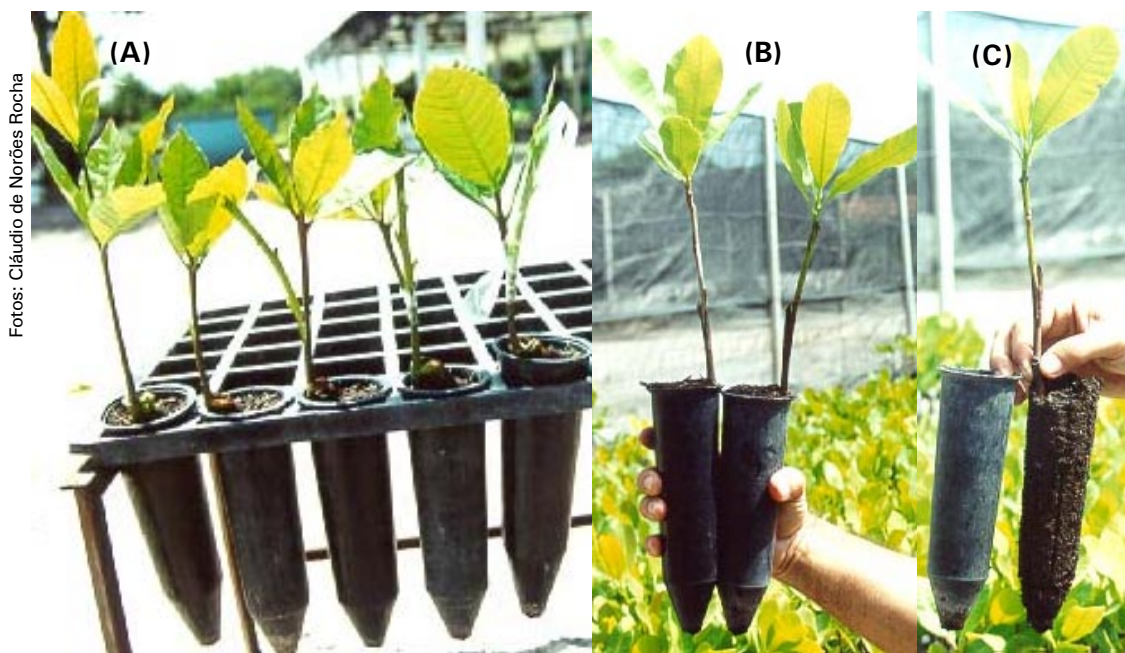
Fig. 2. Detalhe da enxertia do cajueiro anão precoce: (A) por garfagem em fenda lateral em porta-enxertos com 35 dias de idade e, (B) mudas aptas para plantio, com 60 dias depois de enxertadas. Pacajus, CE.1999.
